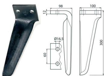
ALPEGO Maschio derecho
